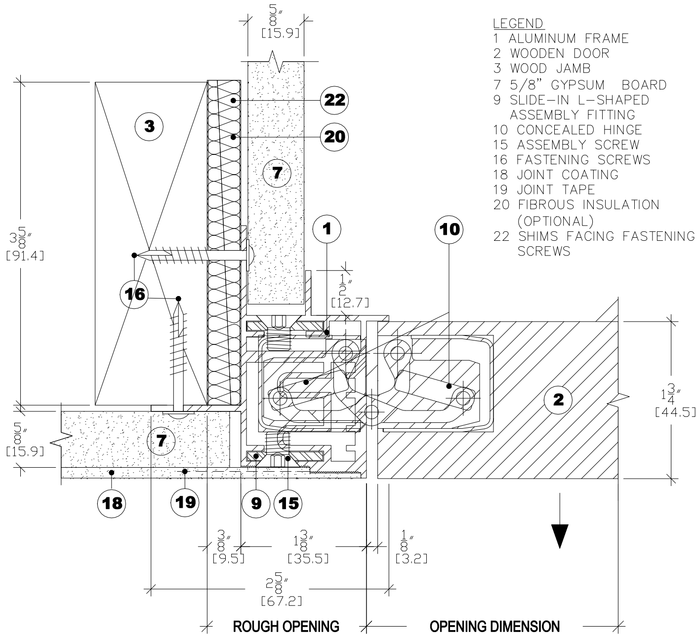
1 JAMB (HINGE SIDE) ACTUAL DIMENSIONS
