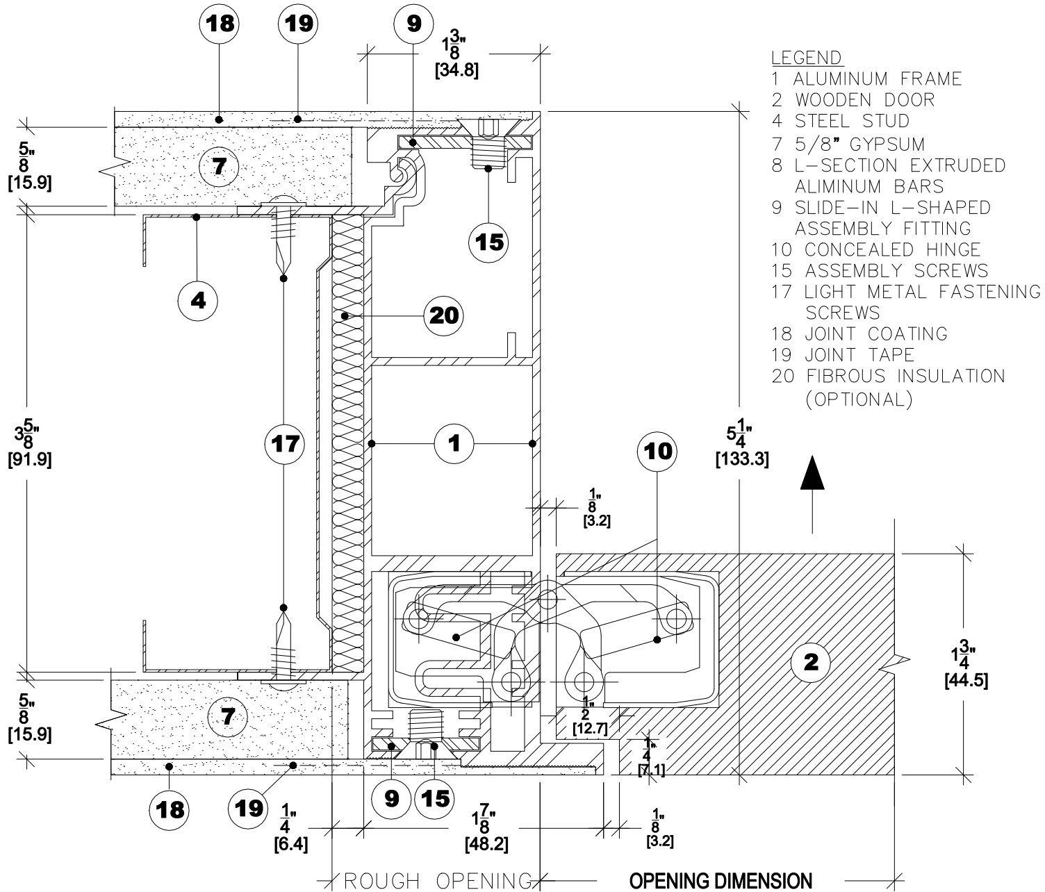
1 JAMB (HINGE SIDE) ACTUAL DIMENSIONS
