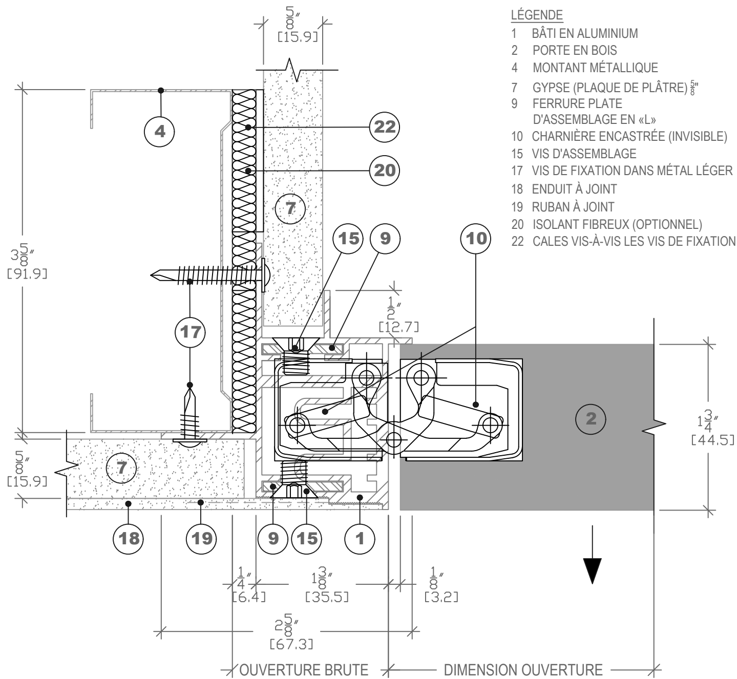
1 JAMBAGE CÔTÉ CHARNIÈRE DIMENSIONS RÉELLES
