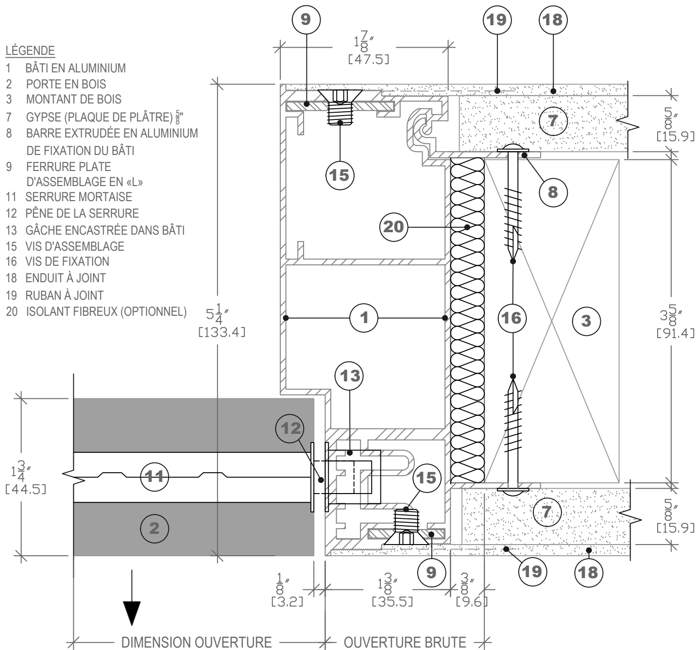
3 JAMBAGE CÔTÉ SERRURE DIMENSIONS RÉELLES
