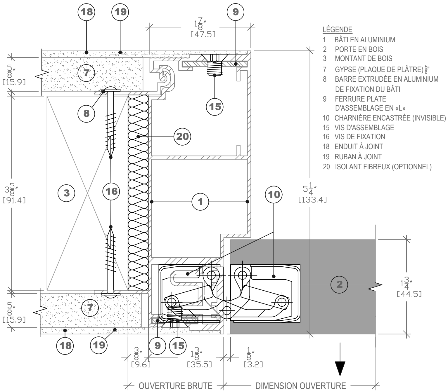
1 JAMBAGE CÔTÉ CHARNIÈRE DIMENSIONS RÉELLES
